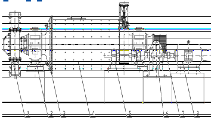
1. 联合给料器 2. 轴承部 3. 进料部 4. 筒体部 5. 传动部 6. 减速机 7. 自料部 8. 电动机
